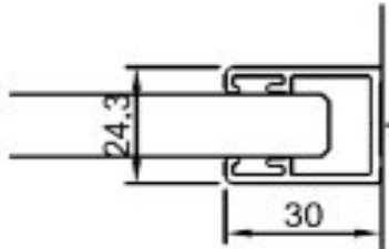
Profilé U
