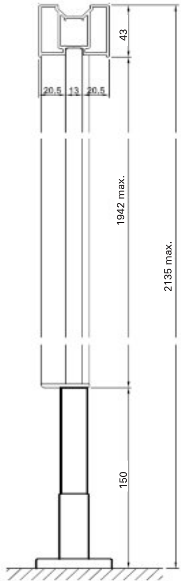
Coupe configuration standard
